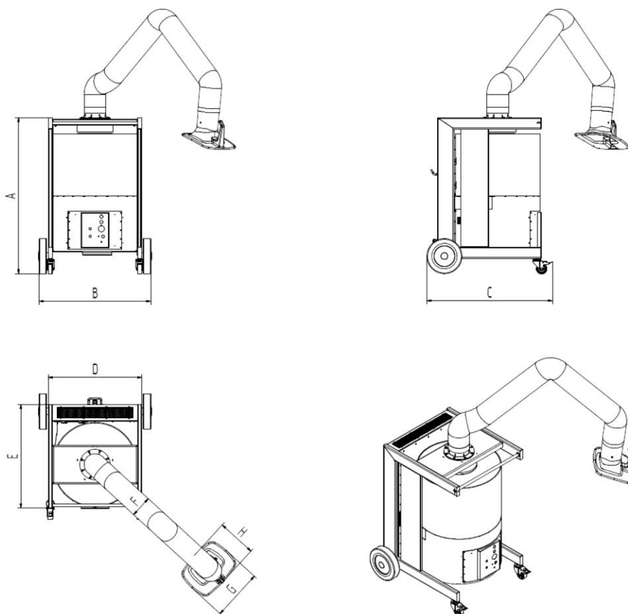
Abb. 15: Maßblatt
